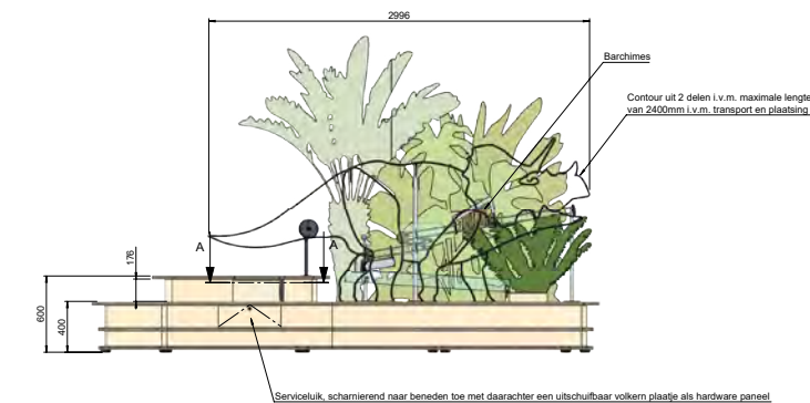
Service-luik, scharnierend naar beneden toe met daarachter een uitschuifbaar volkern plaatje als hardware paneel
