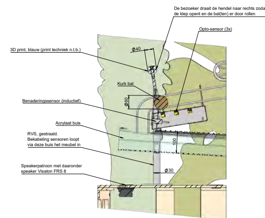
SECTION E SCALE 1 :
